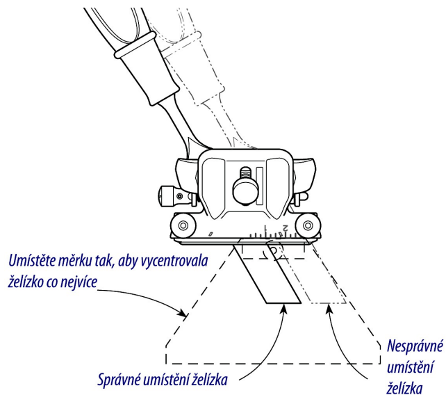
Obr. 7: Želízko vycentrováno pomocí měrky.
