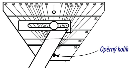
Obr. 6: Nastavení měrky ke zkopírování již existujícího kosého úhlu.
