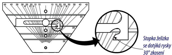
Obr. 4: Nastavení stopky želízka, když je úhel znám
